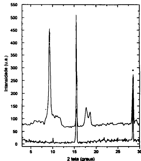
Figura 6. Difratogramas de raios-X dos compostos 1T-TiS 2 (a) e \text{Li}_x(\text{DMF})_y\text{TiS}_2 (b), possíveis contaminantes das fases apresentadas na figura 5.
