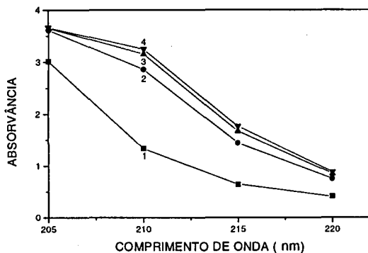
Figura 2. Efeito da concentração de \text{Na}_2\text{SO}_4 no sinal espectrofotométrico de zircônio. Zr: 1254 \text{ mgL}^{-1} ; Meio: \text{HCl} : 2,0 \text{ molL}^{-1} ; 1: Sem adição de \text{Na}_2\text{SO}_4 ; 2: \text{Na}_2\text{SO}_4 0,042 \text{ molL}^{-1} ; 3: \text{Na}_2\text{SO}_4 0,094 \text{ molL}^{-1} ; 4: \text{Na}_2\text{SO}_4 0,145 \text{ molL}^{-1} .
