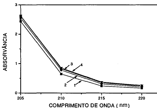
Figura 3. Efeito da concentração de \text{Na}_2\text{SO}_4 no sinal espectrofotométrico de háfnio. Hf: 1891 \text{ mgL}^{-1} ; Meio: \text{HCl} : 2,0 \text{ molL}^{-1} ; 1: Sem adição de \text{Na}_2\text{SO}_4 ; 2: \text{Na}_2\text{SO}_4 0,044 \text{ molL}^{-1} ; 3: \text{Na}_2\text{SO}_4 0,099 \text{ molL}^{-1} ; 4: \text{Na}_2\text{SO}_4 0,150 \text{ molL}^{-1} .
