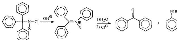
Figura 2. Rearranjo de Stieglitz.
