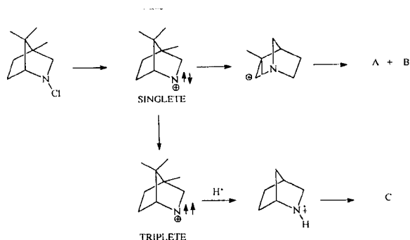
Figura 6. Esquema mecanístico da solvólise do 4,4,7,2-cloro-2-azabíciclo [2.2.1]heptano.
