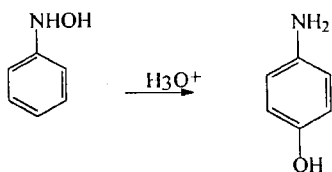
Figura 8. Rearranjo de Bamberg.
