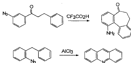
Figura 20. Ciclização intramolecular de íons fenil-nitrênio. Formação de anéis fundidos de 6 e 7 membros.
