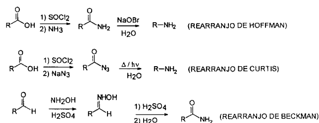
Figura 15. Esquemas sintéticos para os rearranjos de Hoffman, Curtius e Beckman.
