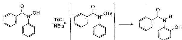
Figura 10. Formação e decomposição de N-tosil-hidroxiclamatos.
