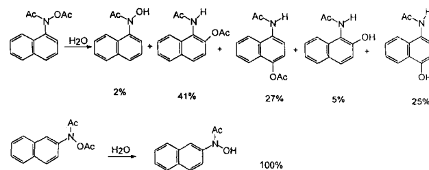
Figura 22. Hidrólise de derivados N-acetoxi-N-naftil-acetamida.
