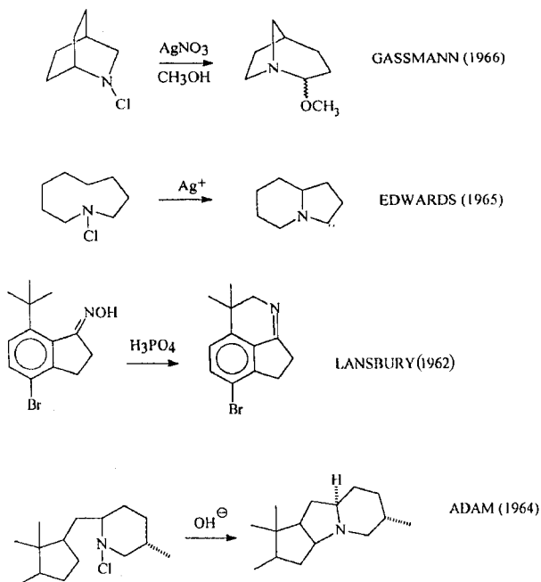
Figura 3. Primeiros resultados sobre solvólise de N-cloro-aminas e formação íons nitrênio.
