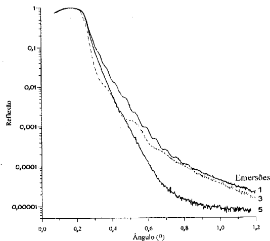
Figura 2. Curvas de reflexão especular de raios x das camadas delgadas de SnO 2 preparadas com uma, três e cinco emersões.
