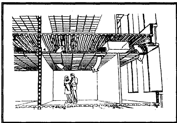
Figura 1. Transporte de poluentes nos dutos de ar condicionado. 1: poluentes presentes em uma sala entram na saída de ar (retorno de ar); 2: o ar de outra sala entra no mesmo retorno misturando-se o ar dessas áreas; 3: o ar misturado, após passar pelo ar condicionado, é insuflado para diferentes salas; 4: uma divisória física evita a distribuição para outras máquinas de ar condicionado.
