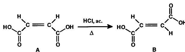
Figura 1. Reacción de isomerización del ácido maleico a ácido fumárico, catalizada por un ácido mineral.
