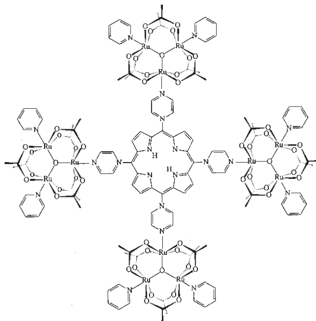
Figura 7. Estrutura de um sistema contendo clusters ligados por porfirina em ponte.
