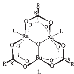
Figura 1. Estrutura esquematizada de [\text{Ru}_3\text{O}(\text{RCO}_2)_6\text{L}_3]^n .
