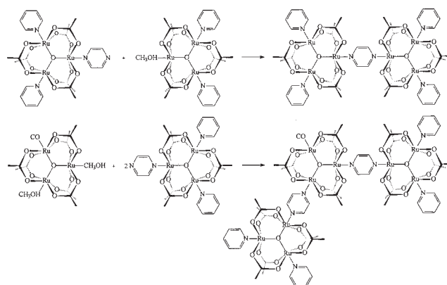
Figura 3. Exemplos de reações de obtenção de dímero e trímero de cluster.
