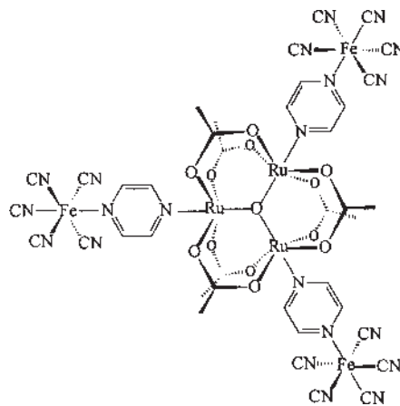
Figura 6. Exemplo de cluster hexanuclear.
