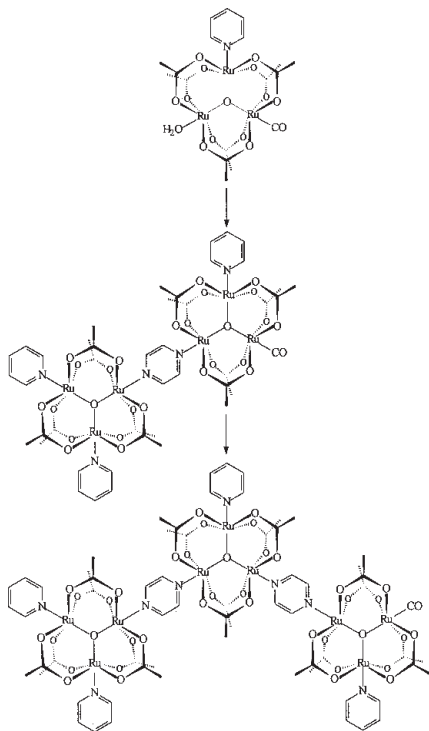
Figura 5. Estruturas esquematizadas de dímeros e trímeros de cluster a partir de um cluster totalmente assimétrico.
