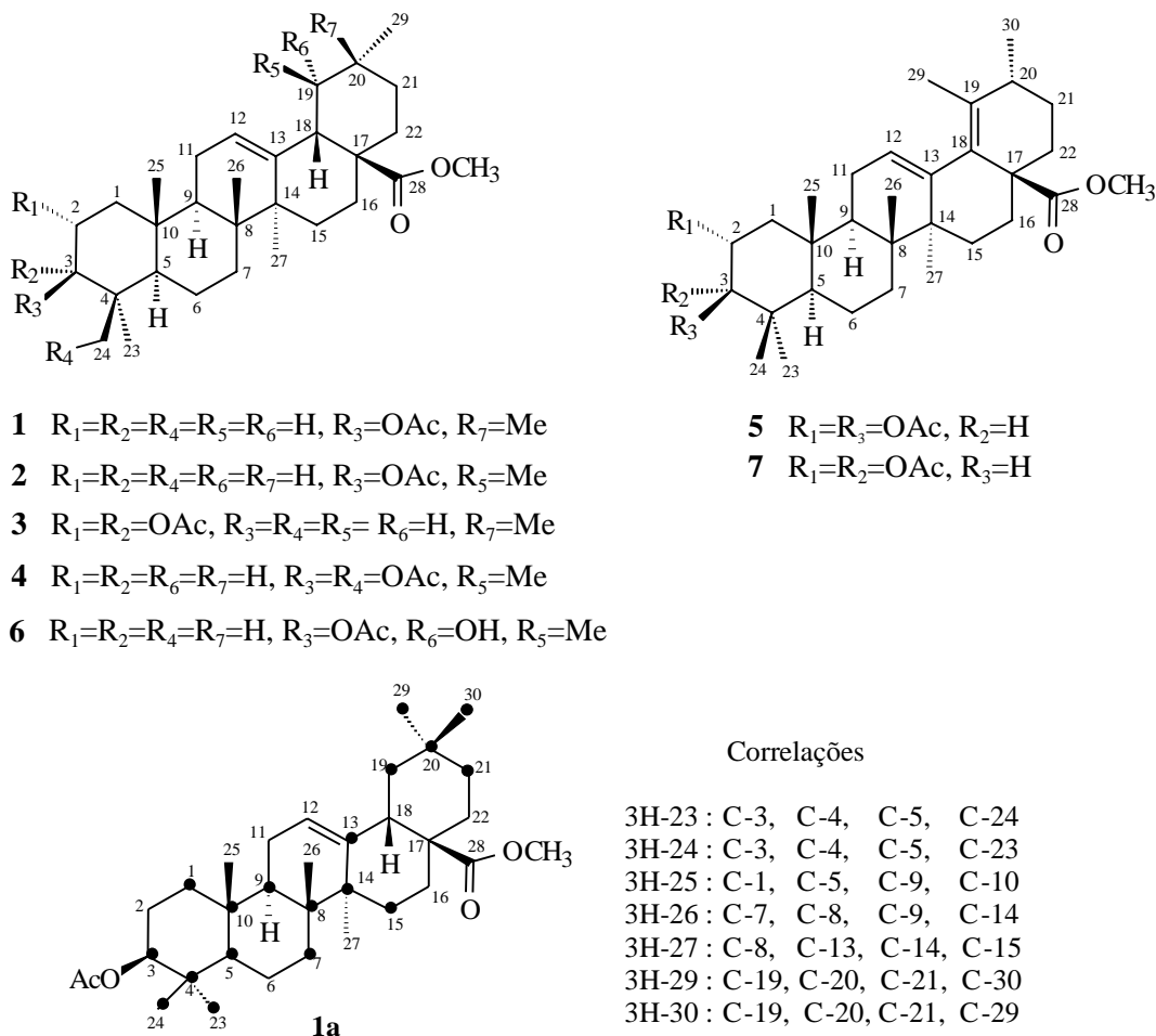
Figura 1. Correlações a longa distância ( ^2J_{CH} e ^3J_{CH} ) entre os hidrogênios metílicos e os respectivos carbonos \alpha e \beta .
