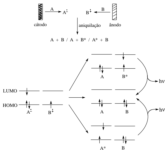
Figura 2. Representação esquemática da quimiluminescência gerada eletroquimicamente, mostrando somente a formação de estados eletronicamente excitados singlete, os quais levam à emissão de quimiluminescência, apesar de estados excitados tripleto também poderem ser formados no processo de aniquilação.
