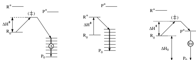
Figura 1. Diagramas de Níveis Energéticos para: A. Reação Térmica Exotérmica, B. Reação Fotoquímica (“foto-energizada”) e C. Reação Quimiluminescente (“químio-energizada”).
