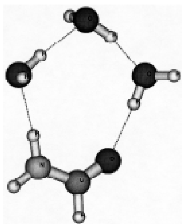
Figura 8. Estrutura molecular para a formamida solvatada por três moléculas de água.
