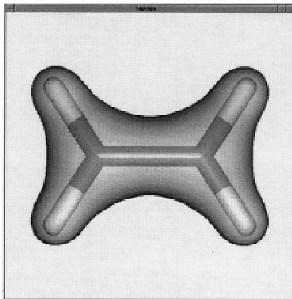
Figura 5. Densidade eletrônica para C_2H_4 , calculada pelo Gamess e visualizada pelo Molden.
