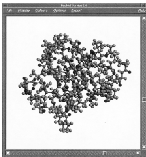
Figura 3. Estrutura da proteína crambin encontrada em sementes e composta por 45 grupos, 752 átomos e 1003 ligações, visualizada pelo pacote gráfico Rasmol.
