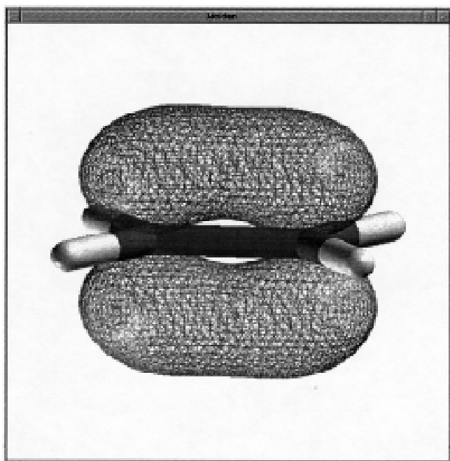
Figura 4. Orbital Molecular para C_2H_4 , obtido pelo Gamess e visualizado pelo Molden.
