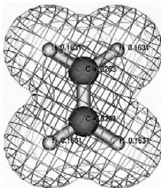
Figura 6. Potencial eletrostático para C_2H_4 , calculado pelo Molden a partir da análise populacional obtida pelo Gamess.
