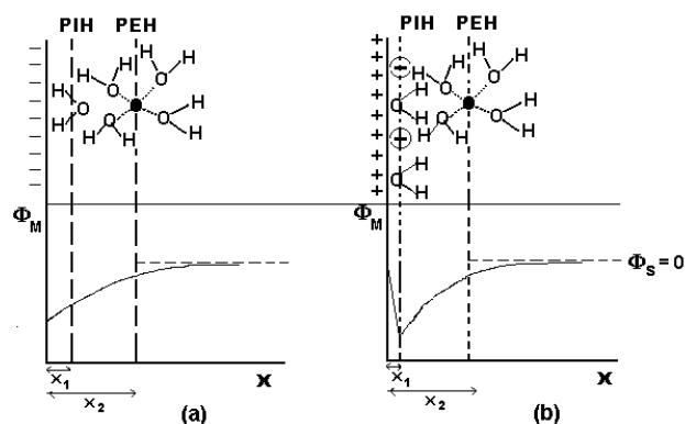
Figura 1. Visão qualitativa da dupla camada elétrica na ausência (a) e presença (b) de adsorção específica. PIH – Plano interno de Helmholtz; PEH – Plano externo de Helmholtz; x_1 – espessura da camada interna; x_2 – espessura da camada externa; ● – cátion; ⊖ – ânion especificamente adsorvido; \Phi_M – potencial no metal; \Phi_s – potencial no meio da solução
