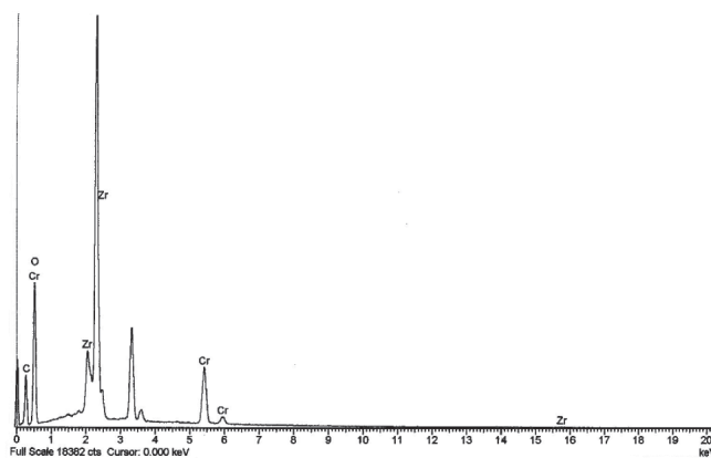
Figura 5. Espectro EDS obtido a partir do compósito Cel/ZrO_2.nH_2O/Cr_2O_7^{2-} (PC)
