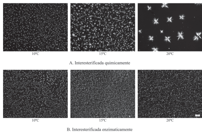
Figura 6. Imagens digitais dos cristais da amostra 6 (óleo de peixe), em função da temperatura (a barra representa 100 \mu\text{m} )
