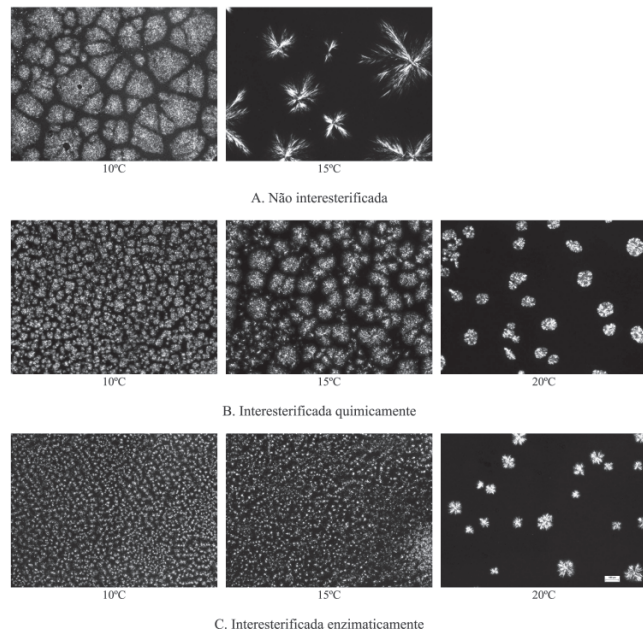
Figura 4. Imagens digitais dos cristais da amostra 4 (palmiste/peixe 40:60), em função da temperatura (a barra representa 100 µm)
