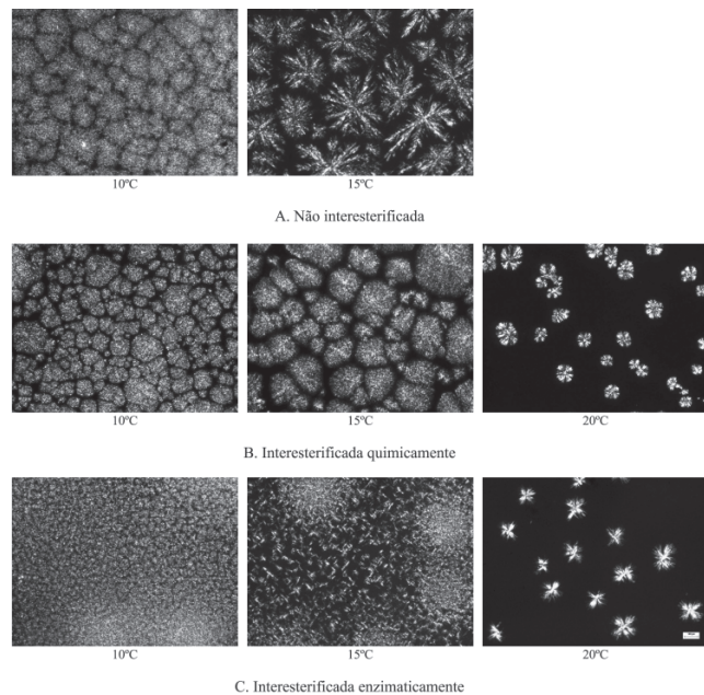
Figura 3. Imagens digitais dos cristais da amostra 3 (palmiste/peixe 60:40), em função da temperatura (a barra representa 100 µm)
