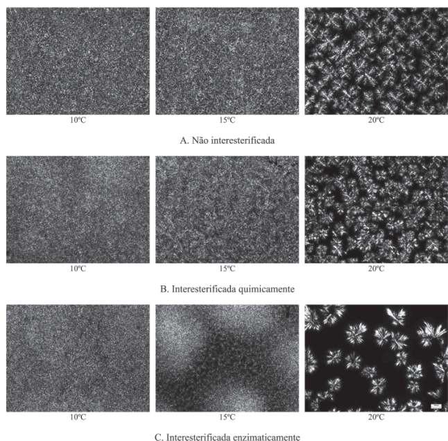
Figura 1. Imagens digitais dos cristais da amostra 1 (gordura de palmiste), em função da temperatura (a barra representa 100 µm)
