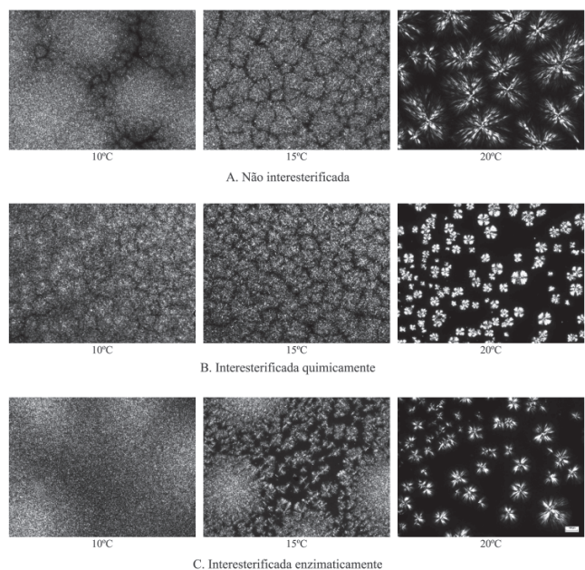
Figura 2. Imagens digitais dos cristais da amostra 2 (palmiste/peixe 80:20), em função da temperatura (a barra representa 100 µm)
