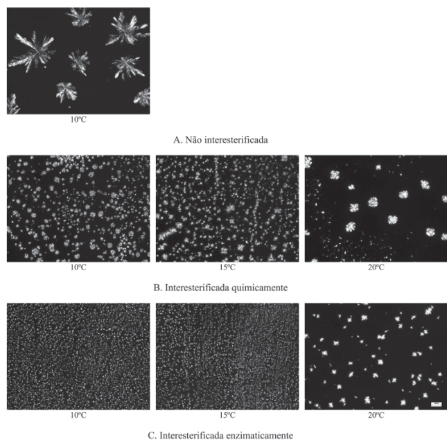
Figura 5. Imagens digitais dos cristais da amostra 5 (palmiste/peixe 20:80), em função da temperatura (a barra representa 100 \mu\text{m} )
