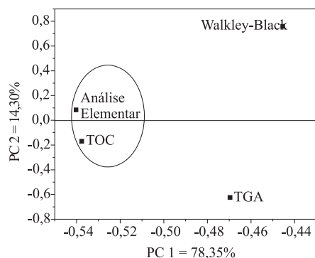
Figura 3. Análise de componentes principais: PC1 x PC2 Loadings correspondentes aos métodos de Walkley-Black, análise elemental, carbono orgânico total (TOC) e análise termogravimétrica (TGA) para determinação de carbono em amostras de solo
