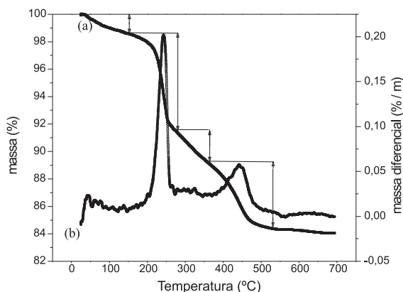
Figura 2. Diagrama termogravimétrico das 4 regiões características no intervalo de 25 a 600 °C: primeira região (< 110 °C); segunda região (150-280 °C); terceira região (270-370 °C) e quarta região (380-530 °C), para a amostra de solo mantido sob sistema de plantio direto (PD), profundidade 0-10 cm, de um Latossolo Vermelho eutroférico (LVef). (a) perda de massa relativa e (b) perda de massa diferencial
