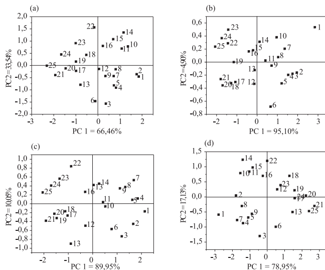
Figura 1. Análise de componentes principais: PC1 x PC2 Scores das metodologias de determinação de carbono por (a) Walkley-Black, (b) Análise elementar, (c) TOC e (d) Walkley-Black, análise elementar e carbono orgânico total (TOC) para determinação do carbono em amostras de solo
