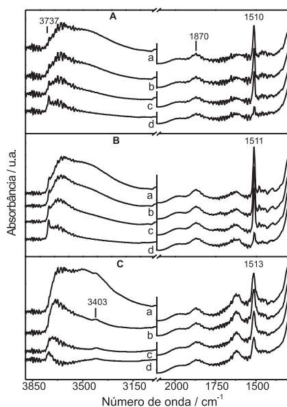
Figura 1. Espectros no infravermelho das sílicas organofuncionalizadas: A) p -anisidina/sílica, B) p -fenitidina/sílica, C) p -fenilenodiamina/sílica; obtidos à temperatura ambiente após tratamento térmico, sob vácuo, nas temperaturas: a) 370, b) 470, c) 570 e d) 670 K
