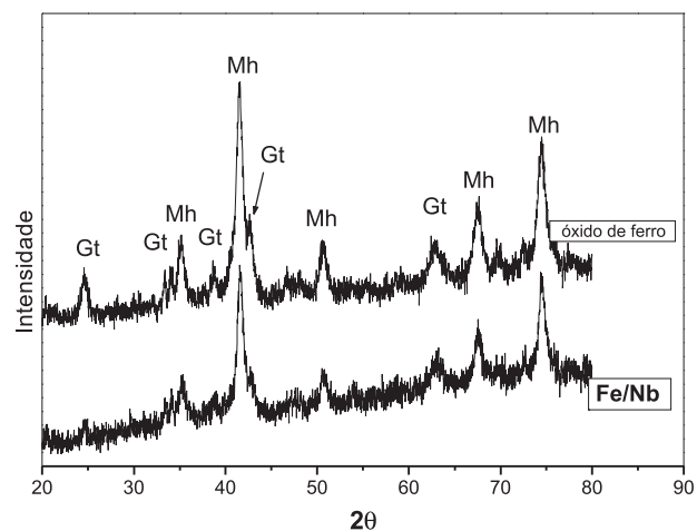
Figura 2. Difratograma de raios-X do óxido de ferro puro e óxido de ferro impregnado em nióbia (Fe/Nb)
