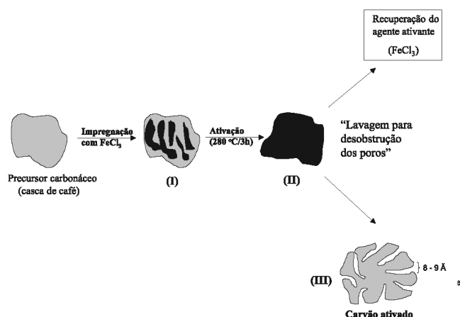
Figura 3. Esquema das etapas de preparação do carvão ativado
