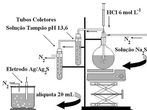
Figura 1. Esquema analítico de extração e fixação de sulfetos
