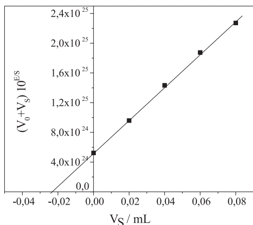
Figura 5. Gráfico de adição de padrão para o teste de recuperação; n = 3
