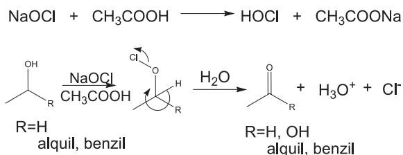
Figura 2. Reação de oxidação de álcoois primários e secundários com hipoclorito de sódio
