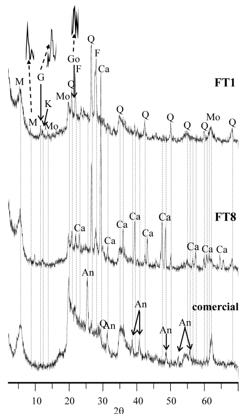
Figura 1. Difratogramas de raios X (Cu Kα) das amostras equatorianas naturais FT1 e FT8 e da argila comercial. Mo: montmorilonita, M: mica, G: gipsita K: caulinita, An: anidrita, Q: quartzo, Go: goethita, F: feldspato e Ca: calcita
