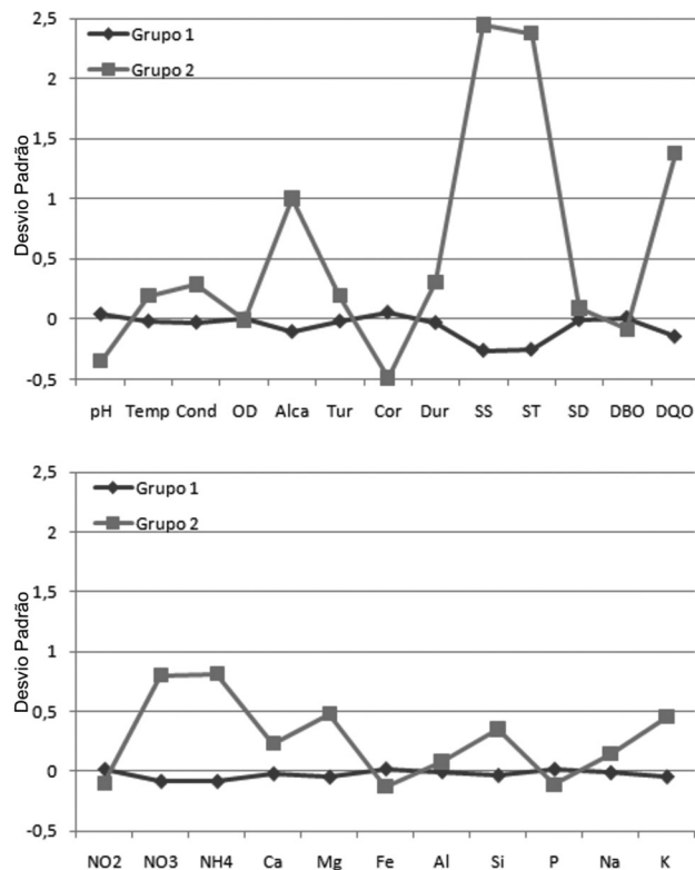
Figura 4. Gráfico resultante da padronização das médias para os parâmetros físico-químicos, compostos nitrogenados e elementos, mostrando as diferenças entre os 2 grupos resultantes da análise agrupamento não-hierárquico
