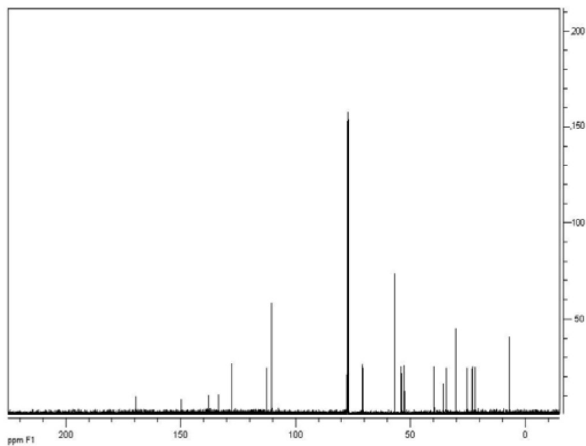
Figura 2S. Espectro de RMN de ^{13}\text{C} de 125 MHz em \text{CDCl}_3 do alcaloide 3
