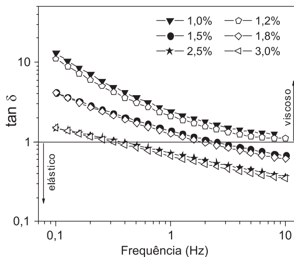
Figura 1S. Efeito da frequência oscilatória e da concentração na tangente de perda das soluções de galactomanana da fava d'anta, a 36 °C
