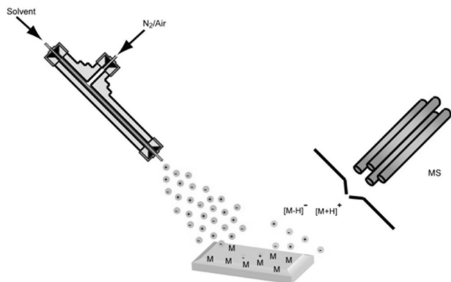
Figura 6. Diagrama esquemático da técnica EASI-MS. Pressão N 2 de 30 bar e vazão do solvente da ordem de 20 \mu\text{L min}^{-1} . Adaptada da ref. 55
