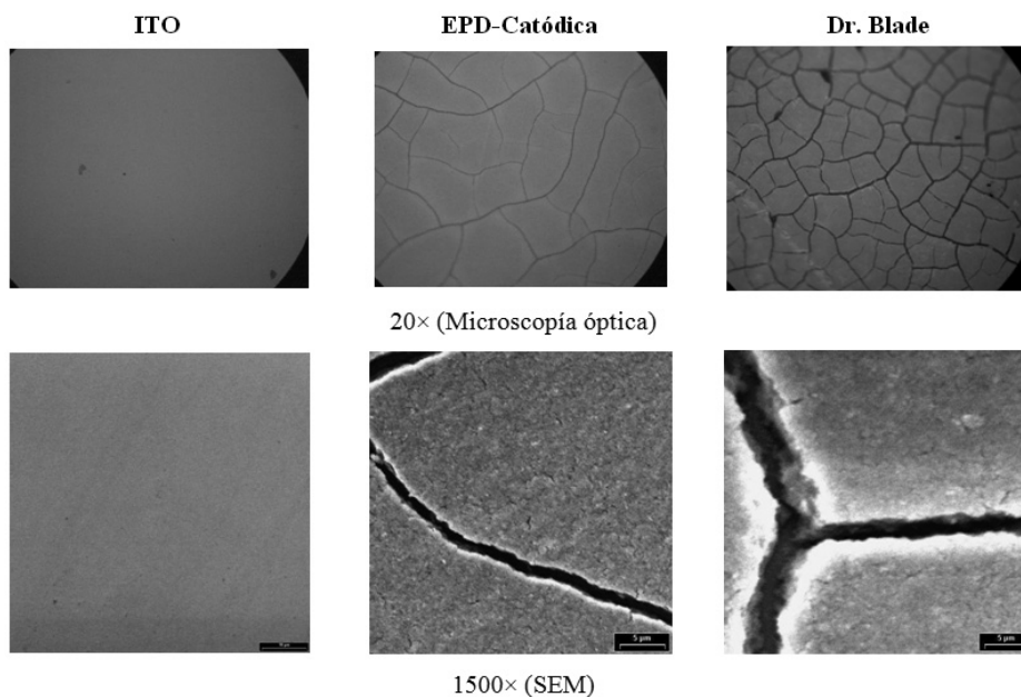
Figura 1S. Micrografías ópticas y de SEM de las películas de \text{TiO}_2 obtenidas
