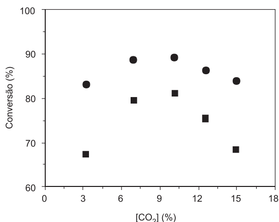
Figura 4. Efeito da concentração de CO 2 na conversão do metano e dióxido de carbono ([CH 4 ] inicial = 8 %). ■ [CO 2 ]; ● [CH 4 ]
