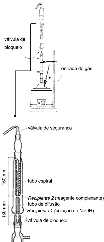
Figura 2. Aparelhagem para a determinação de ditio-carbamatos
