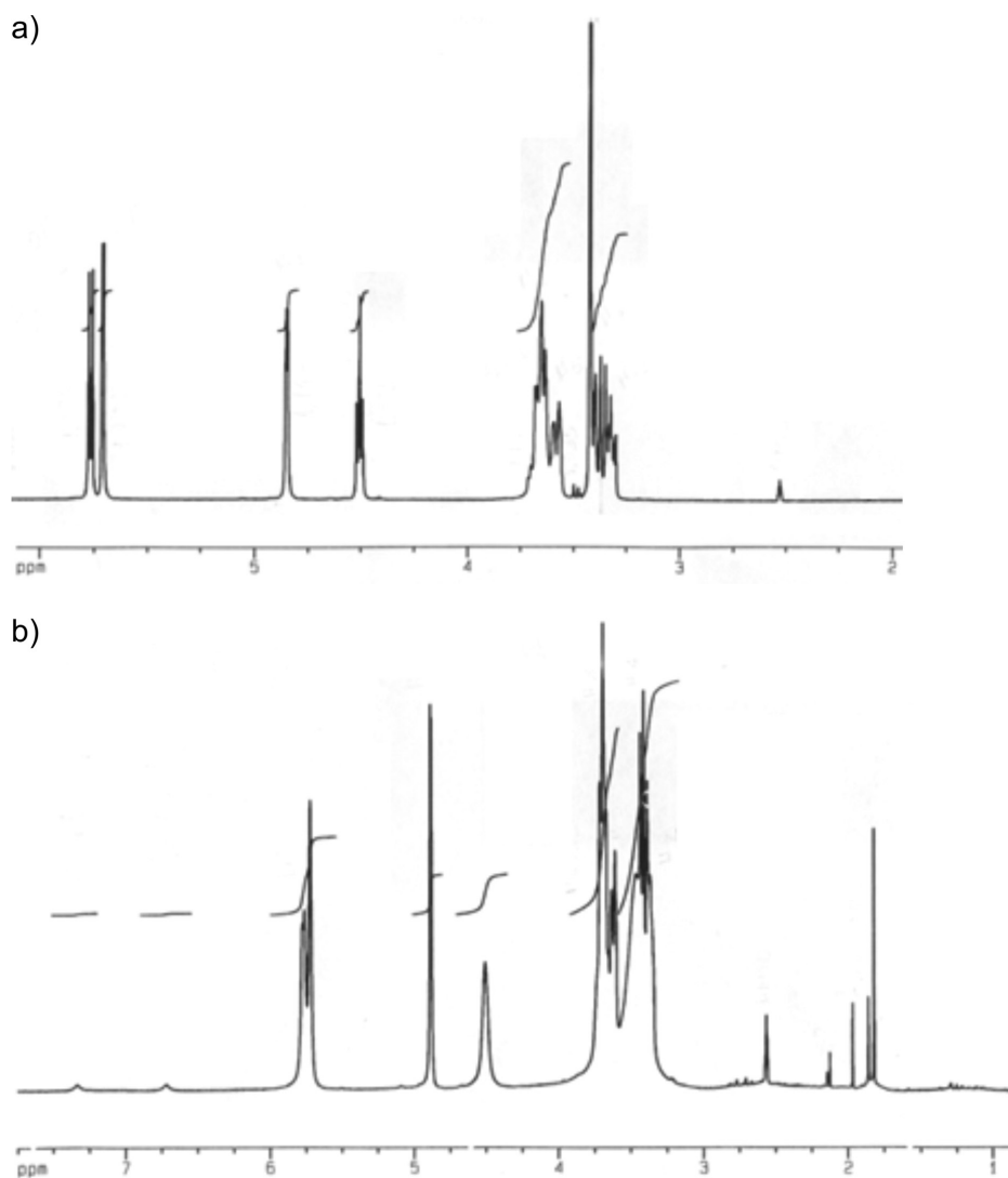
Figura 1S. 1 H RMN de: a) \beta -CD e b) composto de associação ( Rh_2(Cit)_4 - \beta -CD)
