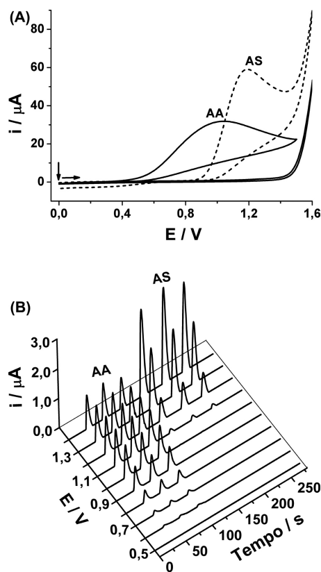
Figura 1. (A) Voltamogramas cíclicos obtidos em meio de tampão HAc/NaAc 0,1 mol \text{L}^{-1} (pH = 4,7) sem e com a adição de 2,0 mmol \text{L}^{-1} de AA ou 2,0 mmol \text{L}^{-1} de AS. Velocidade de varredura de potencial: 50 \text{mV s}^{-1} ; incremento de potencial: 5 \text{mV} . (B) Amperogramas obtidos usando o sistema FIA-MPA na injeção de 60 \mu\text{mol L}^{-1} de AA e 100 \mu\text{mol L}^{-1} de AS. Vazão: 3,0 \text{mL min}^{-1} ; volume injetado: 100 \mu\text{L} ; eletrólito: HAc/NaAc 0,1 mol \text{L}^{-1} ; pulsos de potenciais aplicados: 0,5; 0,6; 0,7; 0,8; 0,9; 1,0; 1,1; 1,2; 1,3 e 1,4 V (50 ms cada)
