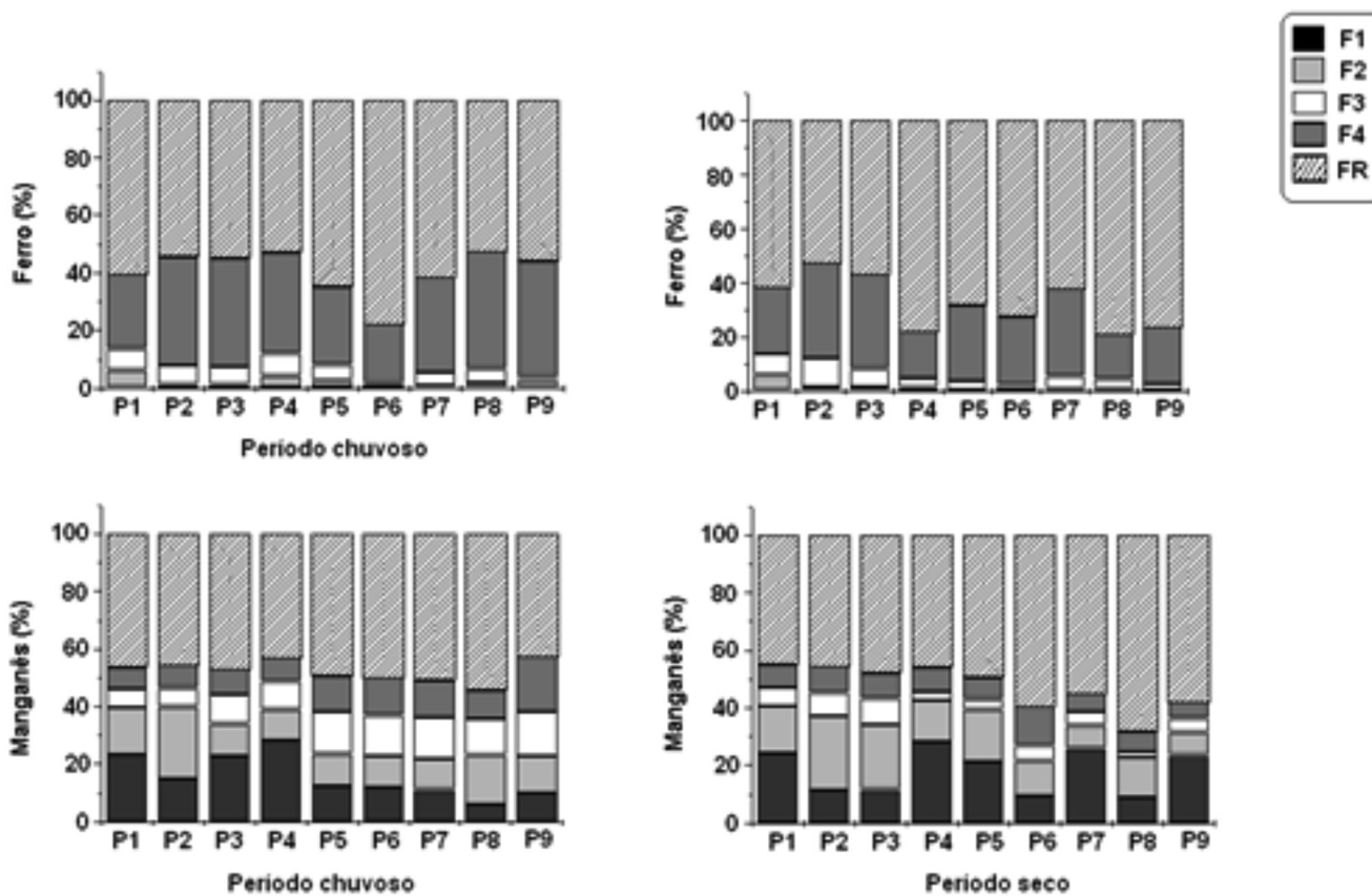
Figura 2S. Percentagens de ferro e manganês distribuídos nas frações do sedimento
