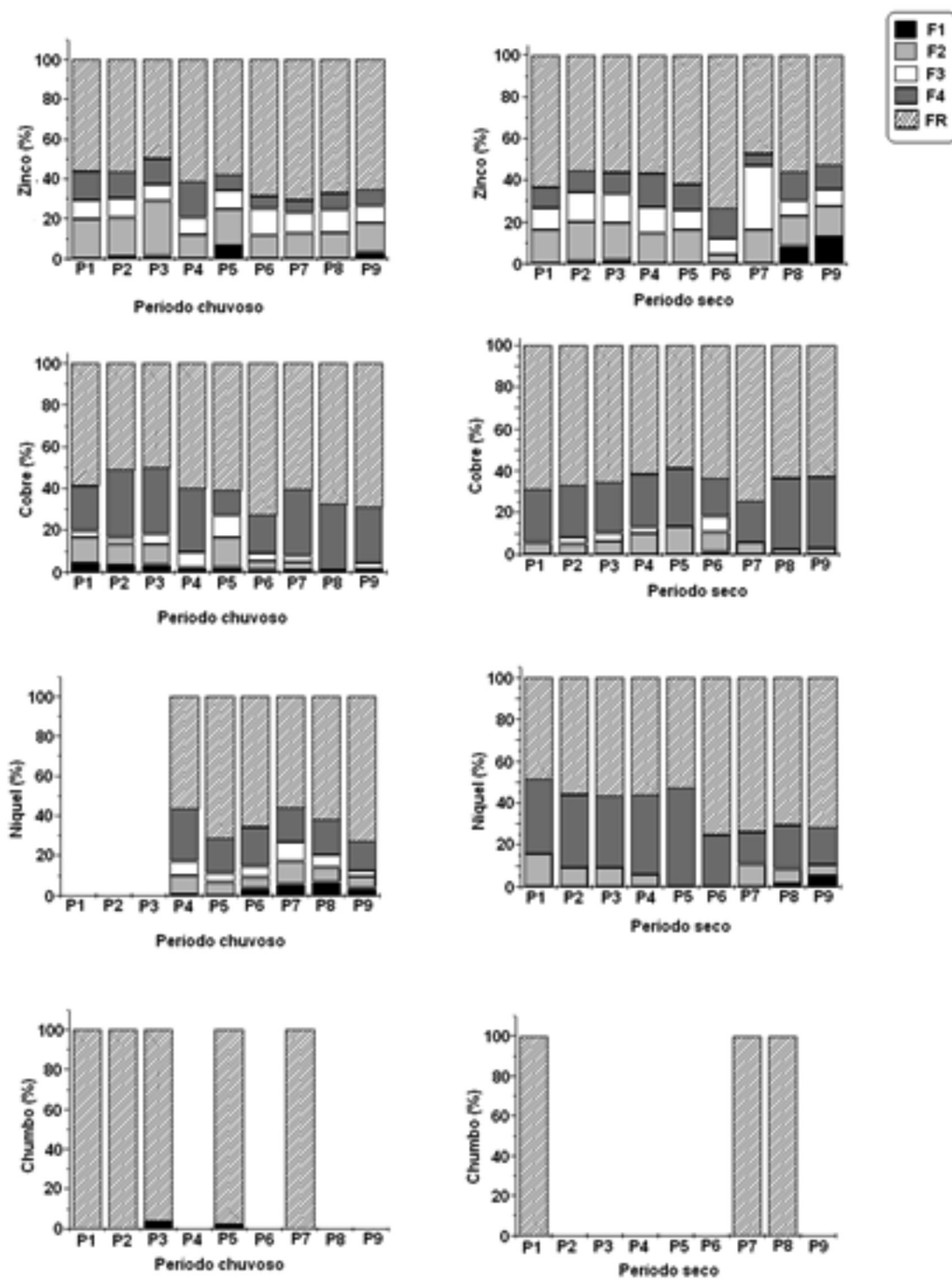
Figura 3S. Percentagens de zinco, cobre, níquel e chumbo distribuídos nas frações do sedimento
