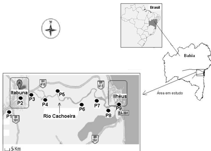
Figura 1S. Área em estudo e os respectivos pontos de coleta
